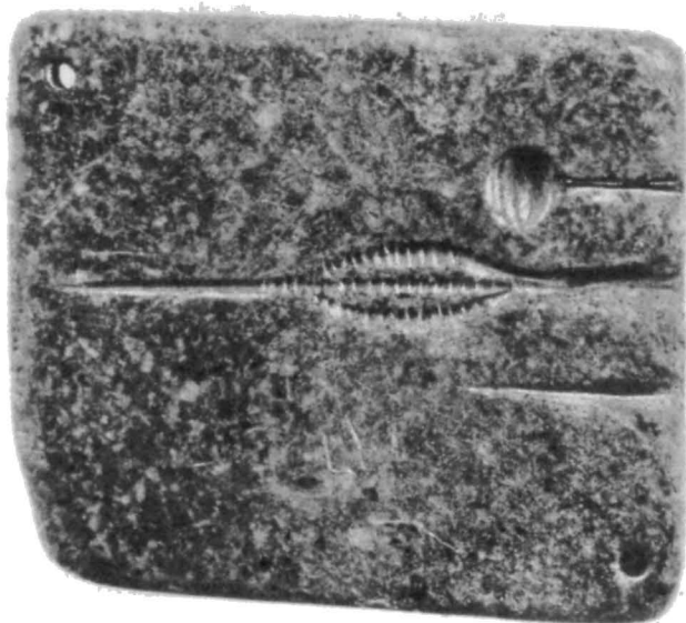
Рис. 7. Литейная форма из Ашшура. Переднеазиатский Музей, Государственные музеи Берлина. Инв. № VA 5870. Фото Музея
